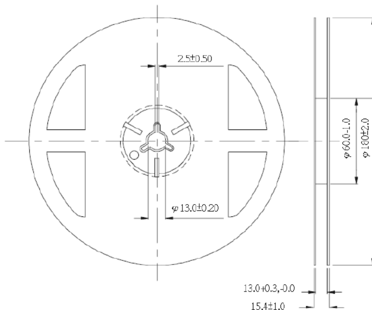
Reel Dimensions
